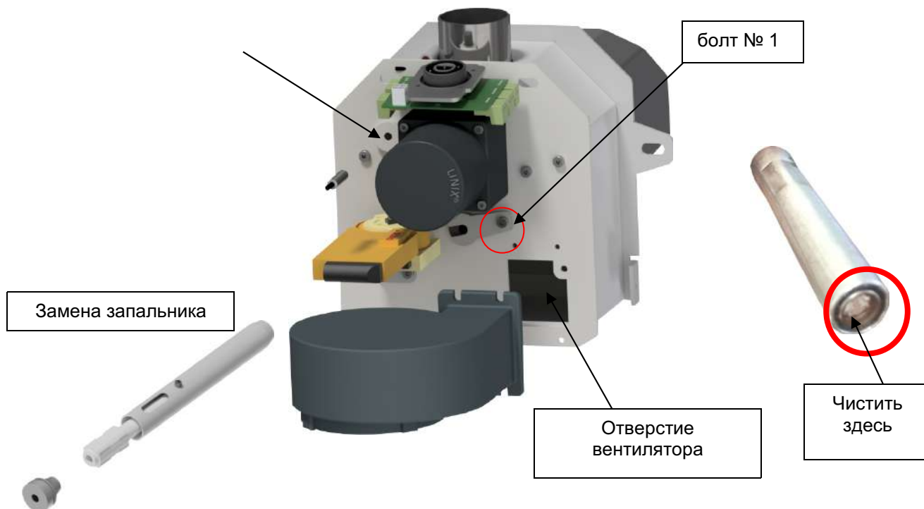
Рисунок 10 - Схема демонтируемых узлов для очистки и ревизии
