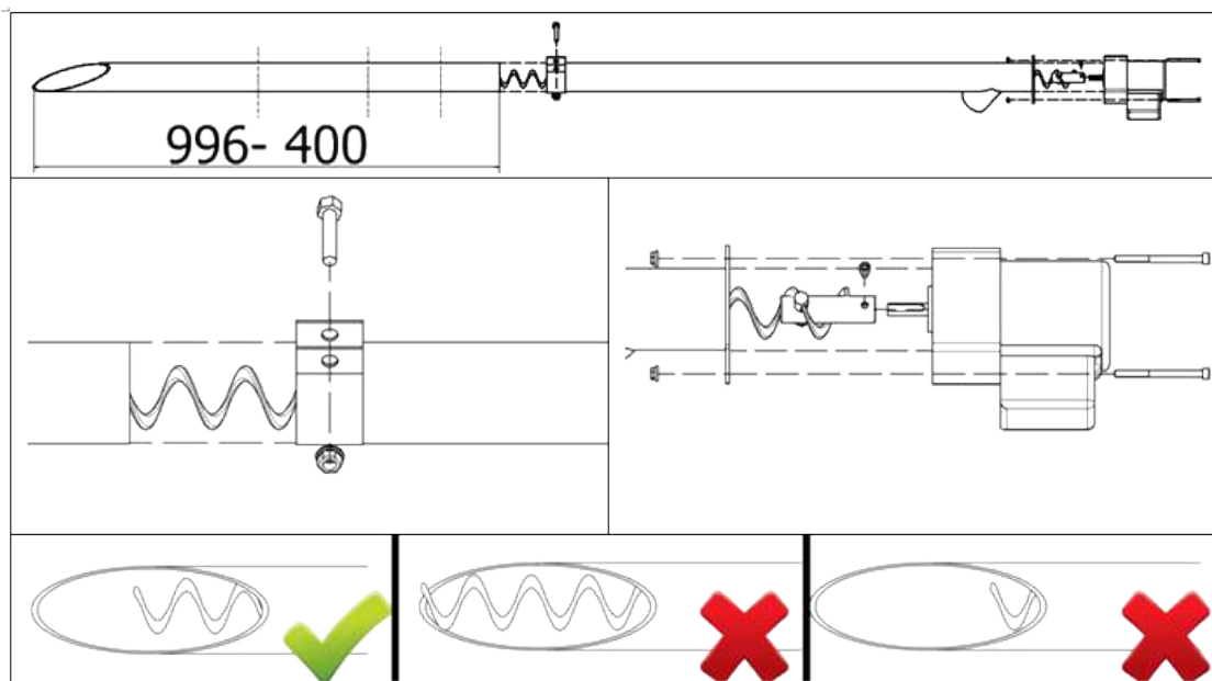
Рисунок 9 – Схема установки винтового подающего устройства в штуцере бункера
