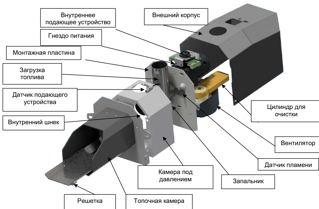
Рисунок 6 – Состав Горелок Lavoro Eco 16-400
