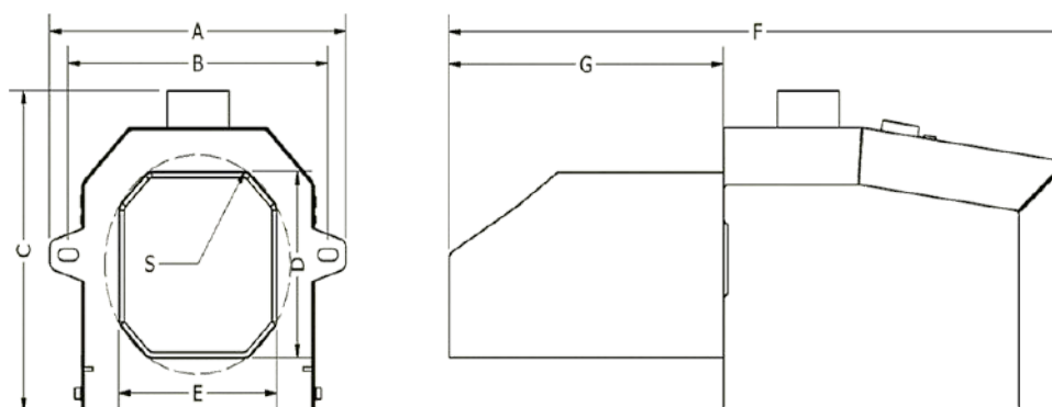
Рисунок 5 – Габаритные и присоединительные размеры Горелок Lavoro Eco 16-400
